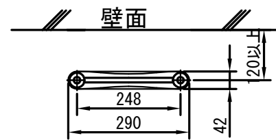
シングルパネルタイプ標準設置例
