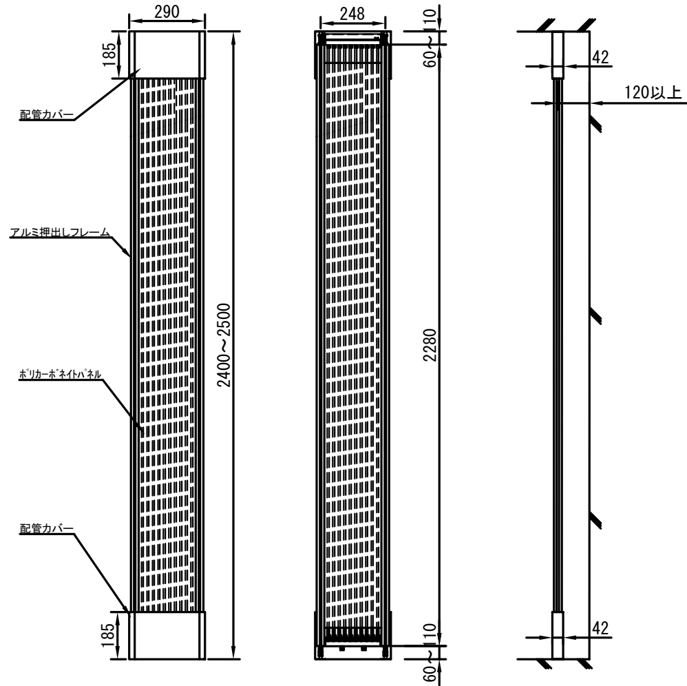
シングルパネルタイプ UR-041AVN2403
