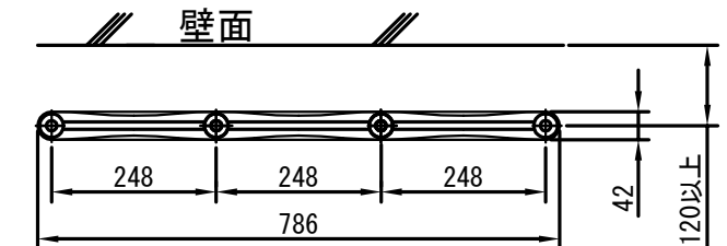
3連タイプ標準設置例
