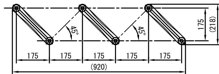
レイヤタイプ設置例
