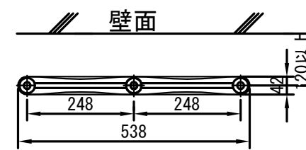
2連タイプ標準設置例
