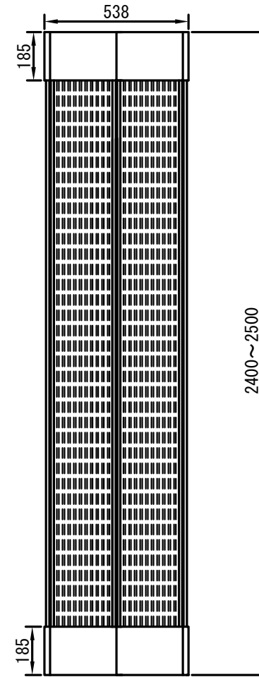
2連パネルタイプ UR-061AVN2406
