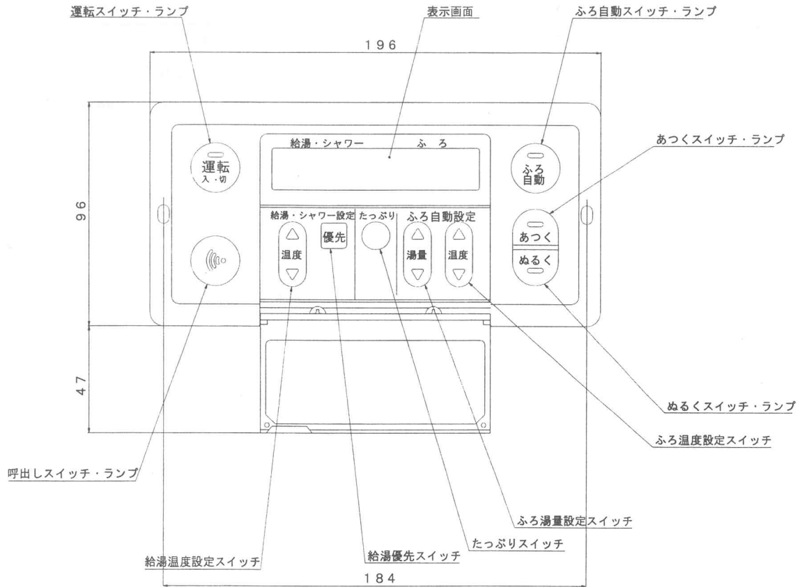
(3) 浴室リモコン外形寸法図
