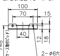
■A部詳細図(S=1/5)
