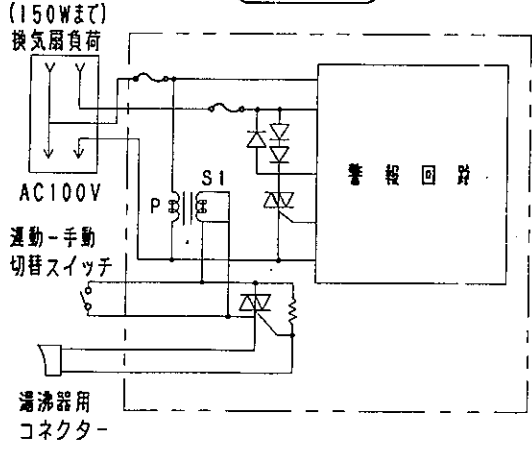
配線図
