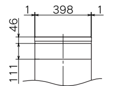
側方排気カバーセットを取り付けた状態
