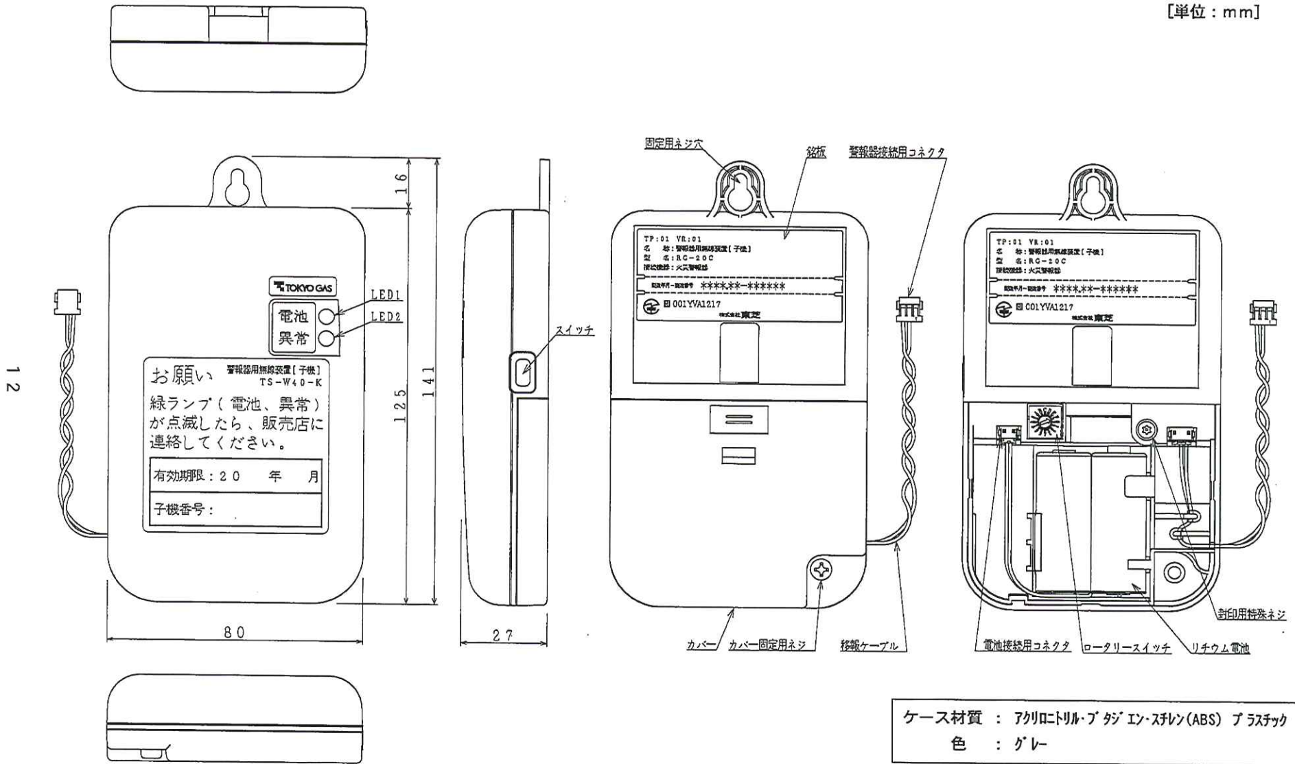
図3.1 TS-W40-K 外観図
