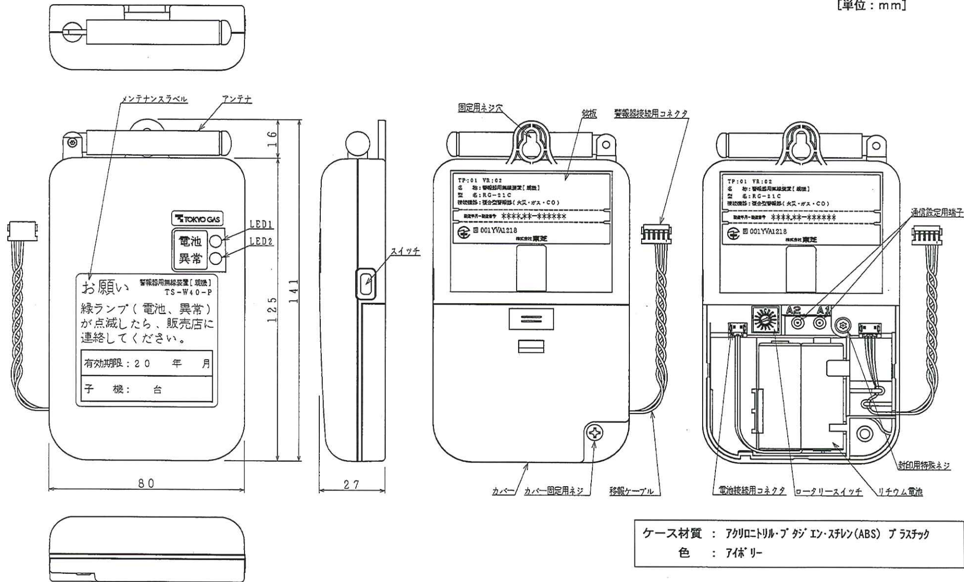
図3.1 TS-W40-P 外観図
