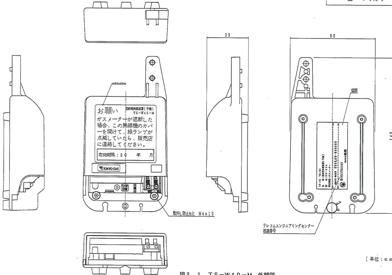
図3.1 TS-W40-M 外觀図
