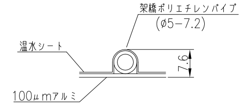
B部拡大図 1/3
