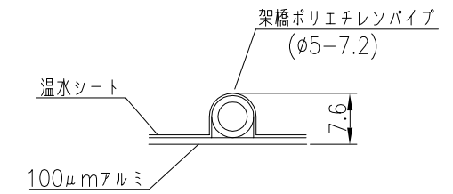
A-A'断面図 1/1
