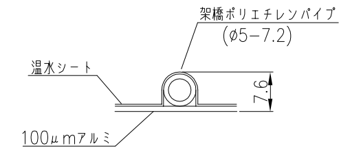
A-A'断面図 1/1
