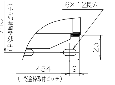
■B部詳細図(S=1/2)
