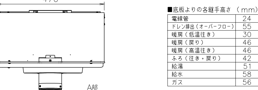
■A部詳細図(S=1/5)
