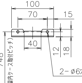
■A部詳細図(S=1/5)
