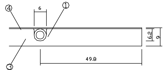
A-A'断面図
