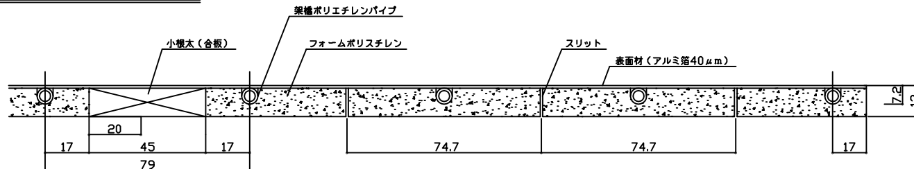
A-A' 断面図 1/1
