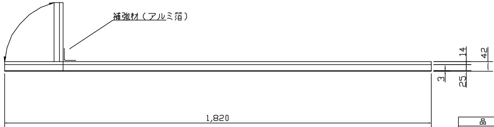
A-A'断面図
