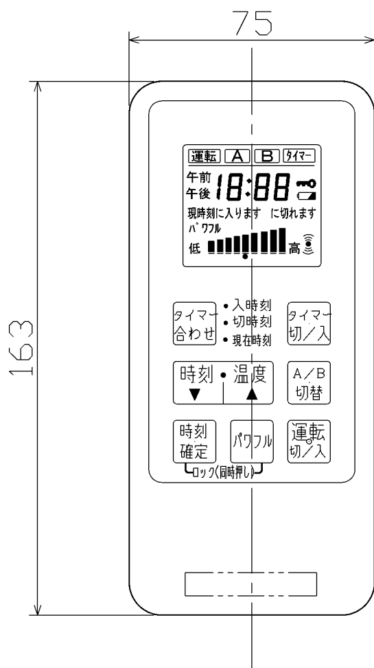
<正面図>
