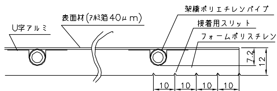
A-A'断面図
