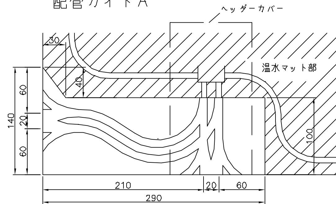
同梱部材 配管ガイド A
