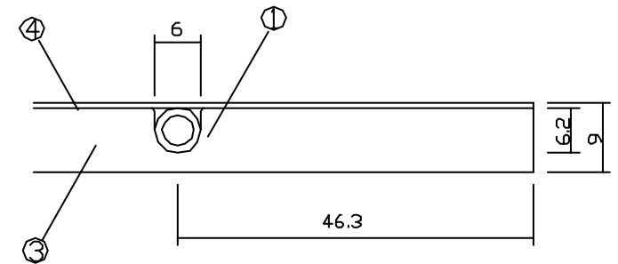
A-A'断面図
