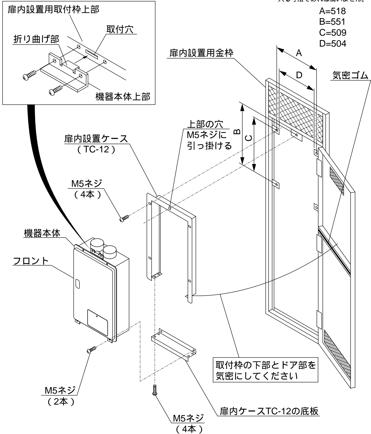
扉内設置用取付枠上部と機器本体上部の取付要領図
