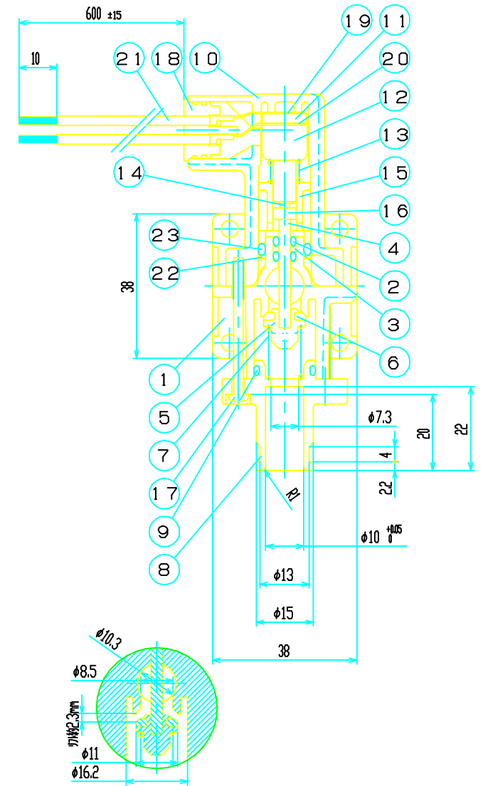
弁全開時詳細図
