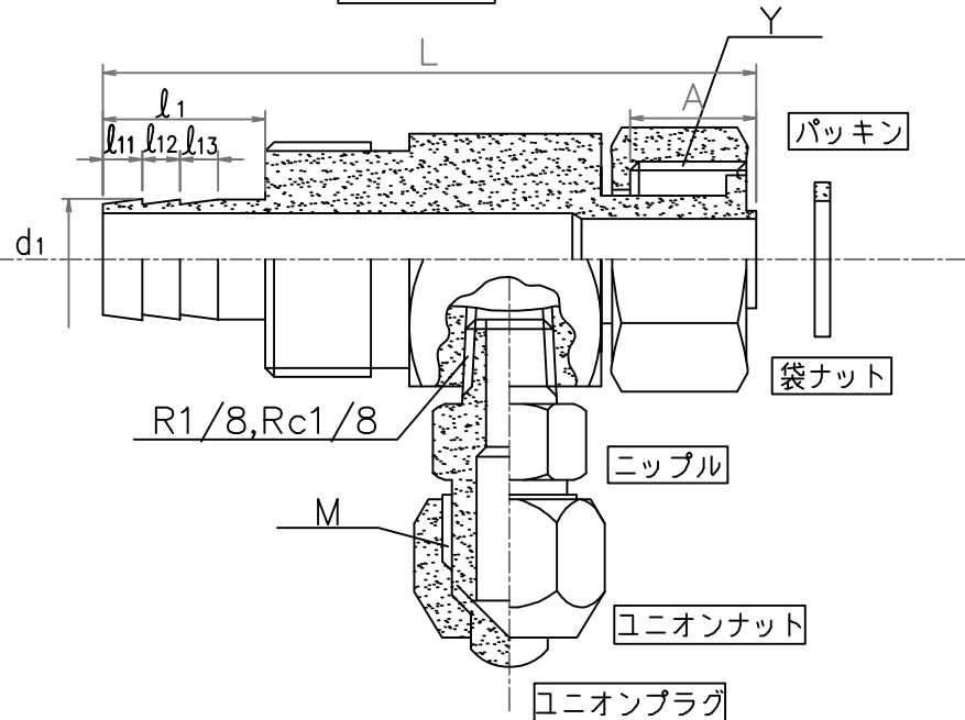
継手本体
