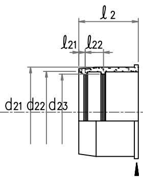
割りリング
