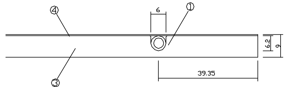
A-A'断面図
