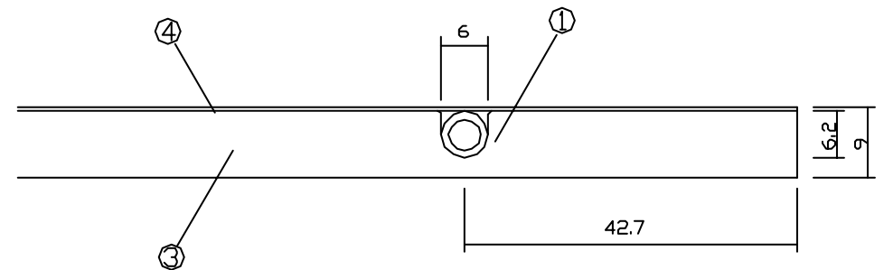
A-A'断面図
