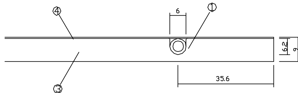
A-A'断面図
