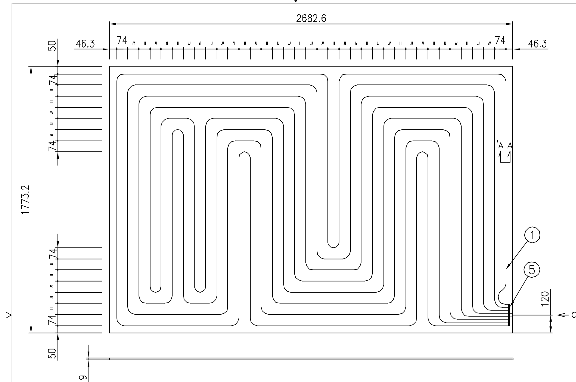
ヘッダー部詳細 1/2 (a方向)
