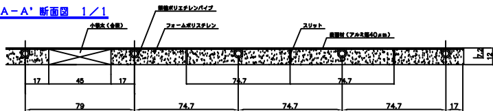
A-A' 断面図 1/1
