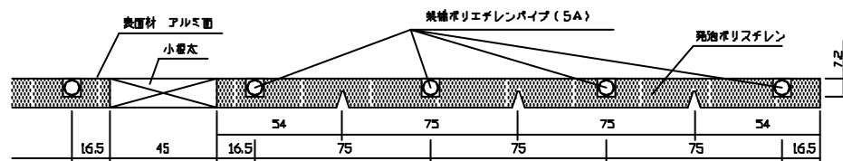
A-A' 断面図
