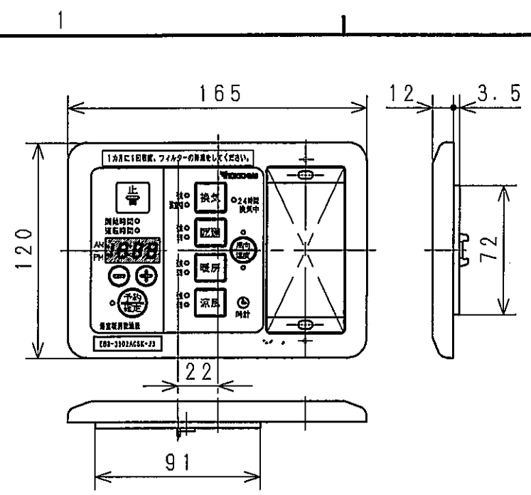
リモコン詳細 (S=1/3)
