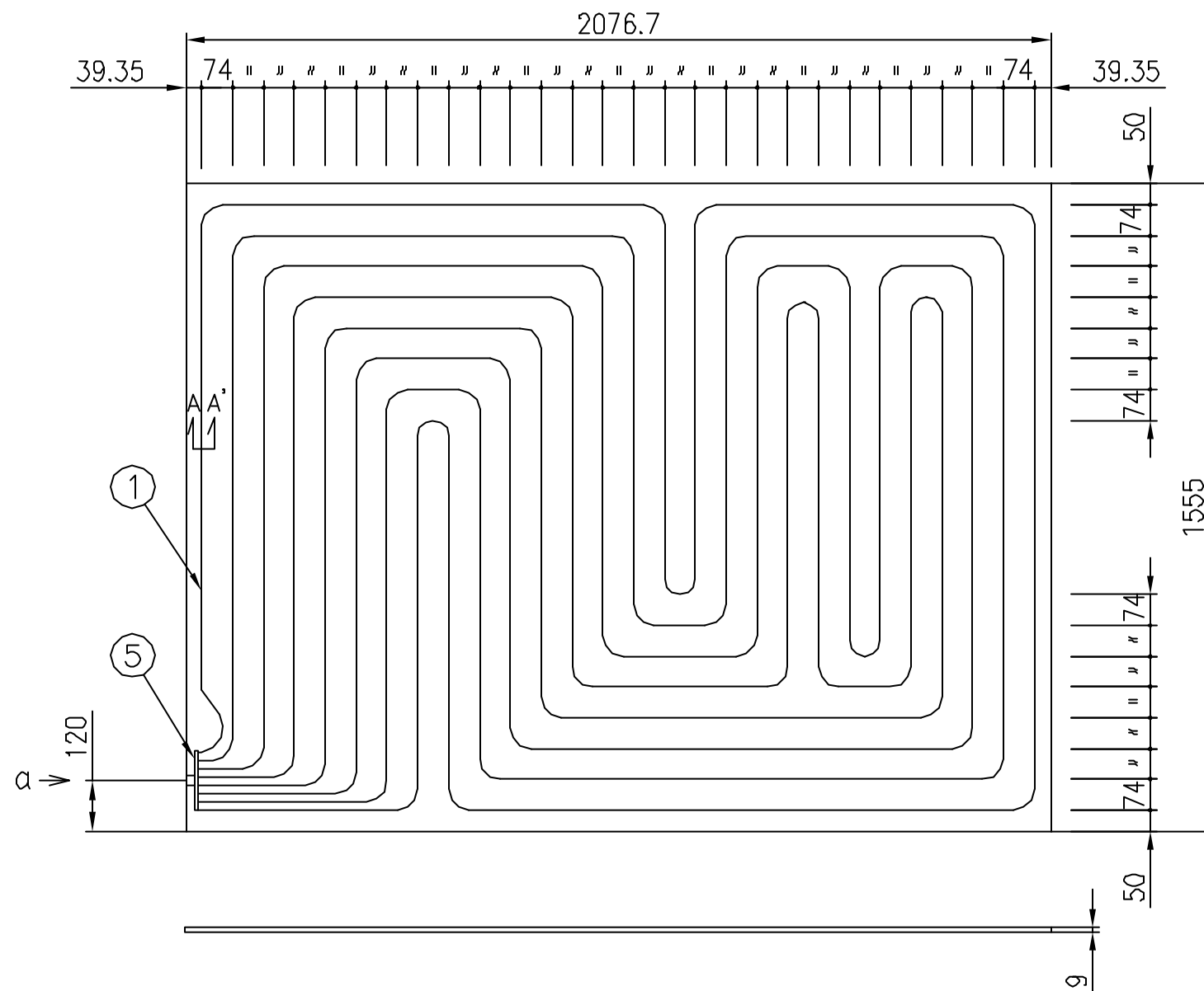
ヘッダー部詳細 1/2 (a方向)
