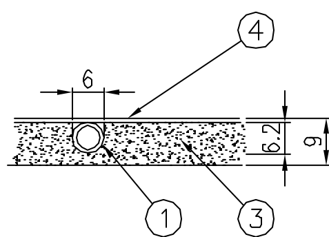
A-A'断面図 1/1
