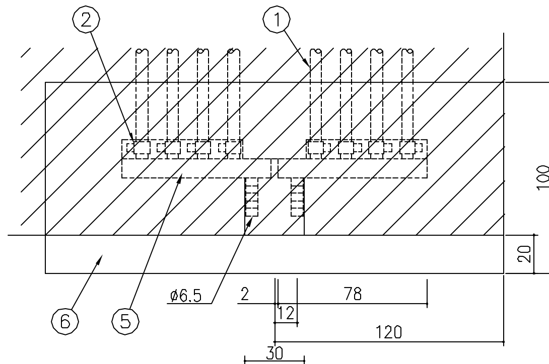
ヘッダー部詳細 1/2 (a方向)
