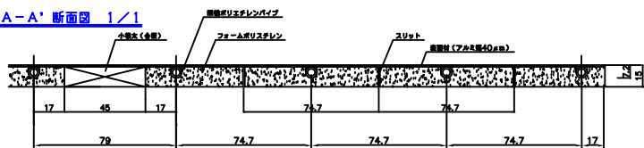
A-A' 断面図 1/1
